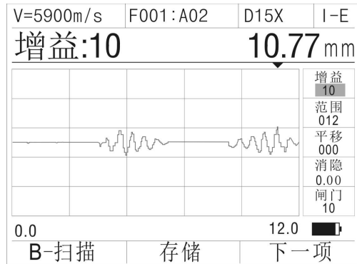
图 3.12 实例图解 1
