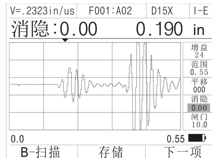
图3.9 消隐前波形
