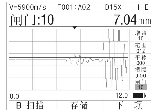
图 3.13 实例图解 2
