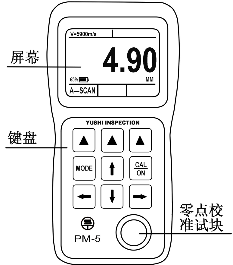
图 1.1 仪器图示
